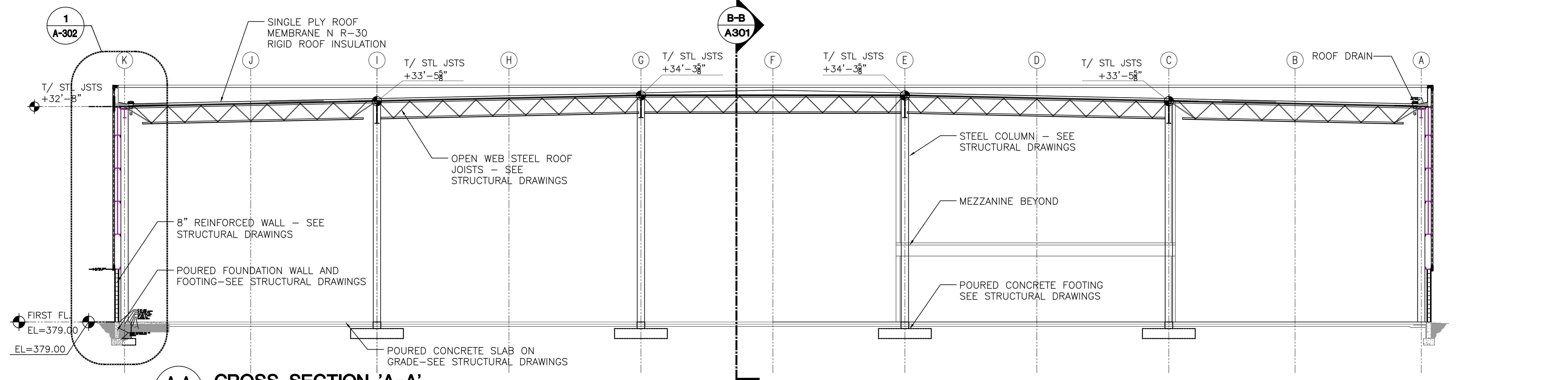
A-A CROSS SECTION 'A-A' SCALE: 1/8" = 1'-0"
