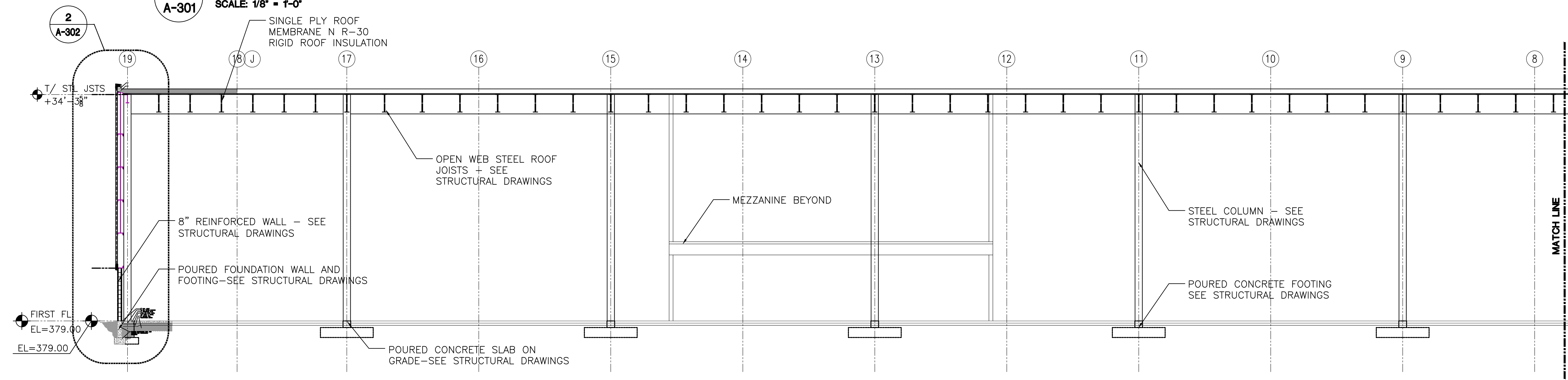
B-B CROSS SECTION 'B-B' SCALE: 1/8" = 1'-0"
